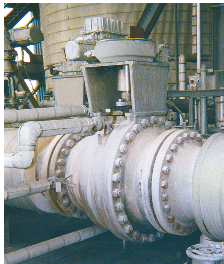
Ces vannes à vapeur à passage intégral NPS 30 (DN 750) sont en service ininterrompu depuis 2002.
