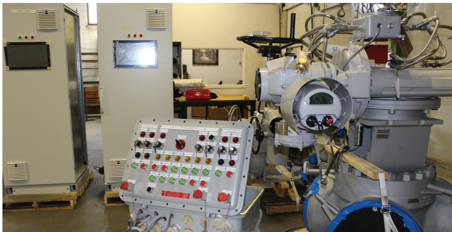
Velan fournit des panneaux de commande locaux fonctionnant de manière autonome et par l'intermédiaire d'un DCS et/ou d'un API. Nos systèmes offrent une gamme complète de verrouillages et de retours d'information pour un fonctionnement en toute sécurité.
