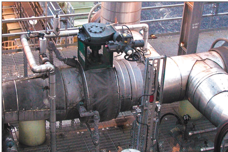
Une grande vanne de vapeur en tête de type NPS 30 (DN 750) installée en 2000 dans une unité de cokéfaction retardée sur la côte du golfe du Mexique aux États-Unis.
