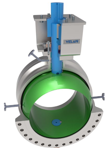
Représenté en position d'ouverture complète
